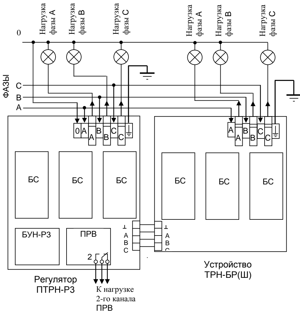
СХЕМА СОЕДИНЕНИЙ
